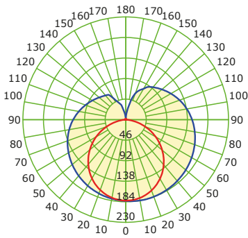
CURVA FOTOMETRICA
